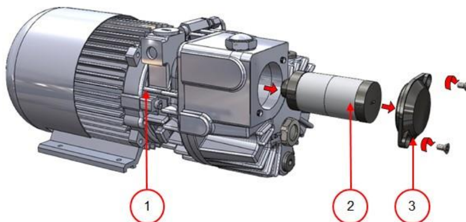
Schéma 11: Remplacement du filtre à échappement d'air (Pompe 9 m 3 /h / 318 cf/h)
