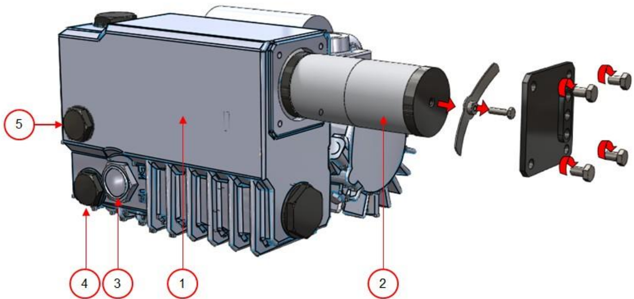
Schéma 5: Aperçu de la pompe (Pompe 19 m 3 /h / 671 cf/h & 25 m 3 /h / 889 cf/h)
