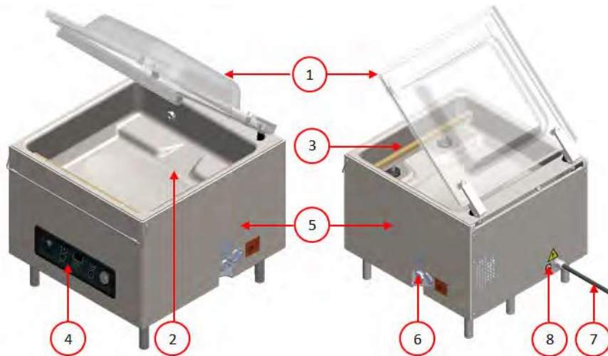
Schéma 1: Aperçu des principaux composants
