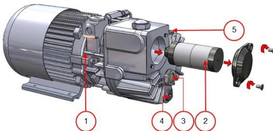
Schéma 4: Aperçu de la pompe (Pompe 9 m 3 /h/ 318 cf/h)
