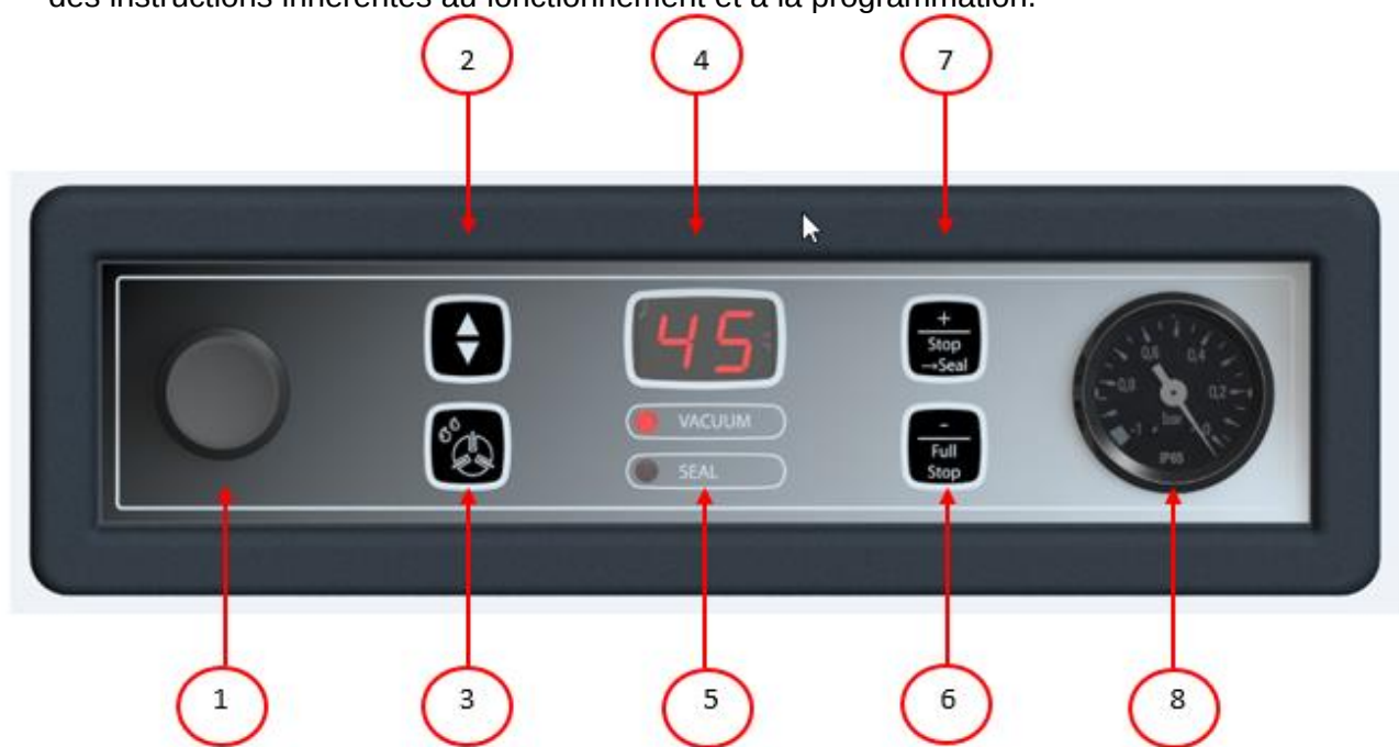
Schéma 7: Panneau de commande du système de commande 1 programme
