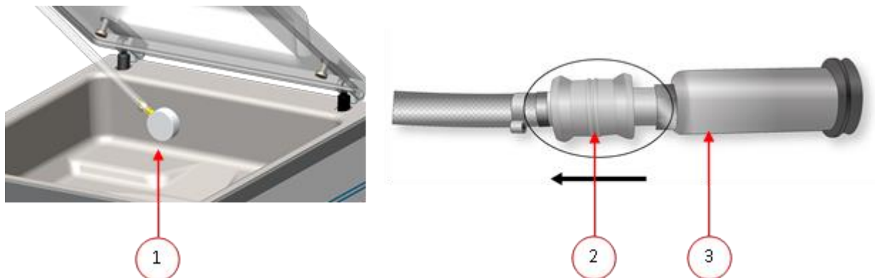
Schéma 8: Kit adaptateur de vide extérieur (Système de commande 1 programme)
