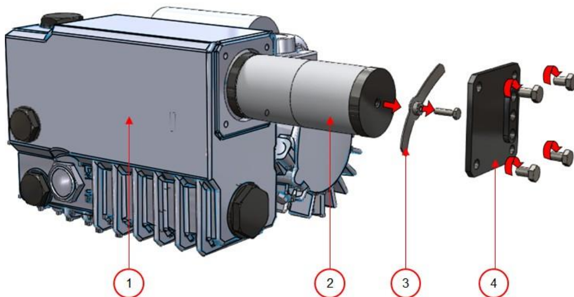
Schéma 12: Remplacement du filtre à échappement d'air (Pompe 16 m 3 /h / 21 m 3 /h)
