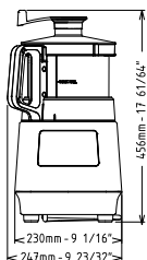
Alzado
