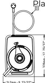
Planta
